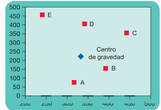
Fig. 5.19. Localización de los puntos y del centro de gravedad representados en la hoja de cálculo. Puedes encontrar la aplicación con esta hoja en el CEO.
