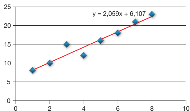
Fig. 2.8. Gráfico de dispersión con recta de regresión en Excel.
