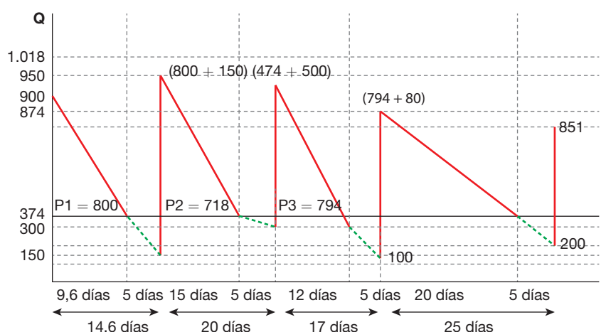
Fig. 4.9. Sistema de reposición mixto.
